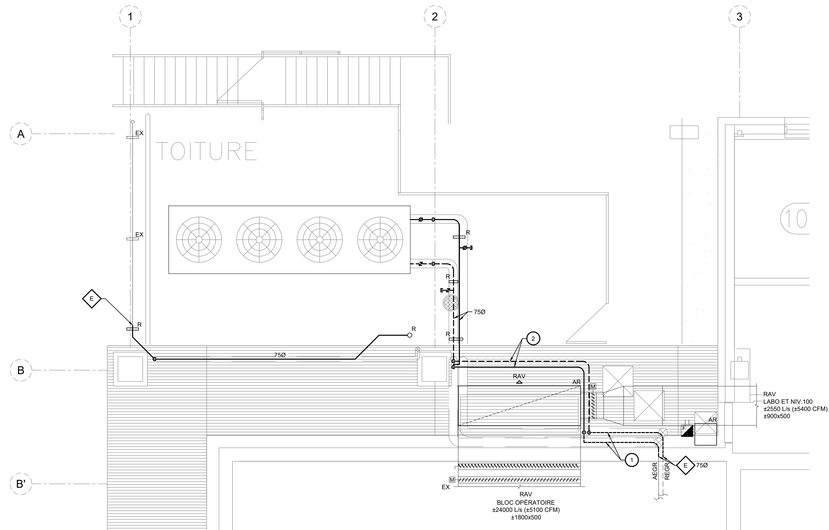
VUE AGRANDIE - TOITURE COIN NORD-OUEST - CONSTRUCTION
