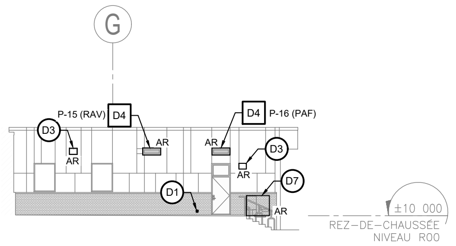
C ÉLÉVATION OUEST PARTIELLE - DÉMOLITION ÉCHELLE: 1:200
