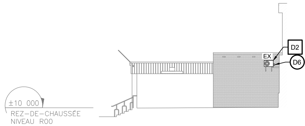
D ÉLÉVATION EST PARTIELLE - DÉMOLITION ÉCHELLE: 1:200
