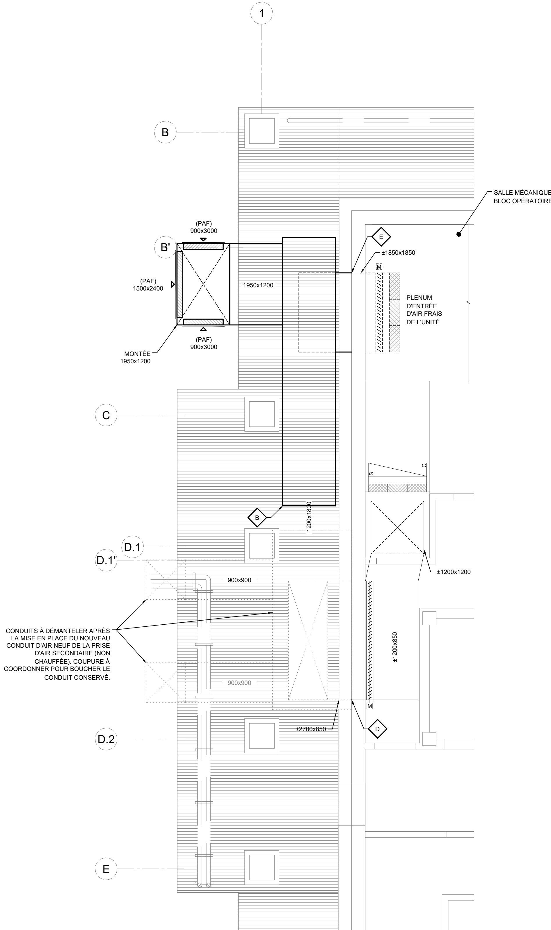
VUE AGRANDIE - TOITURE OUEST - PRISE D'AIR FRAIS BLOC OPÉRATEIRE - TEMPORAIRE #2
