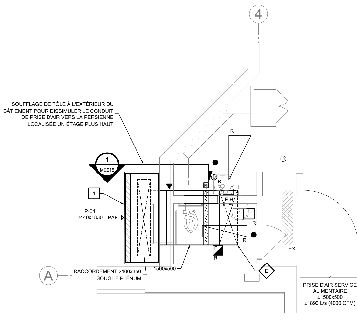
VUE AGRANDIE - PRISE D'AIR SERVICE ALIMENTAIRE - CONSTRUCTION
