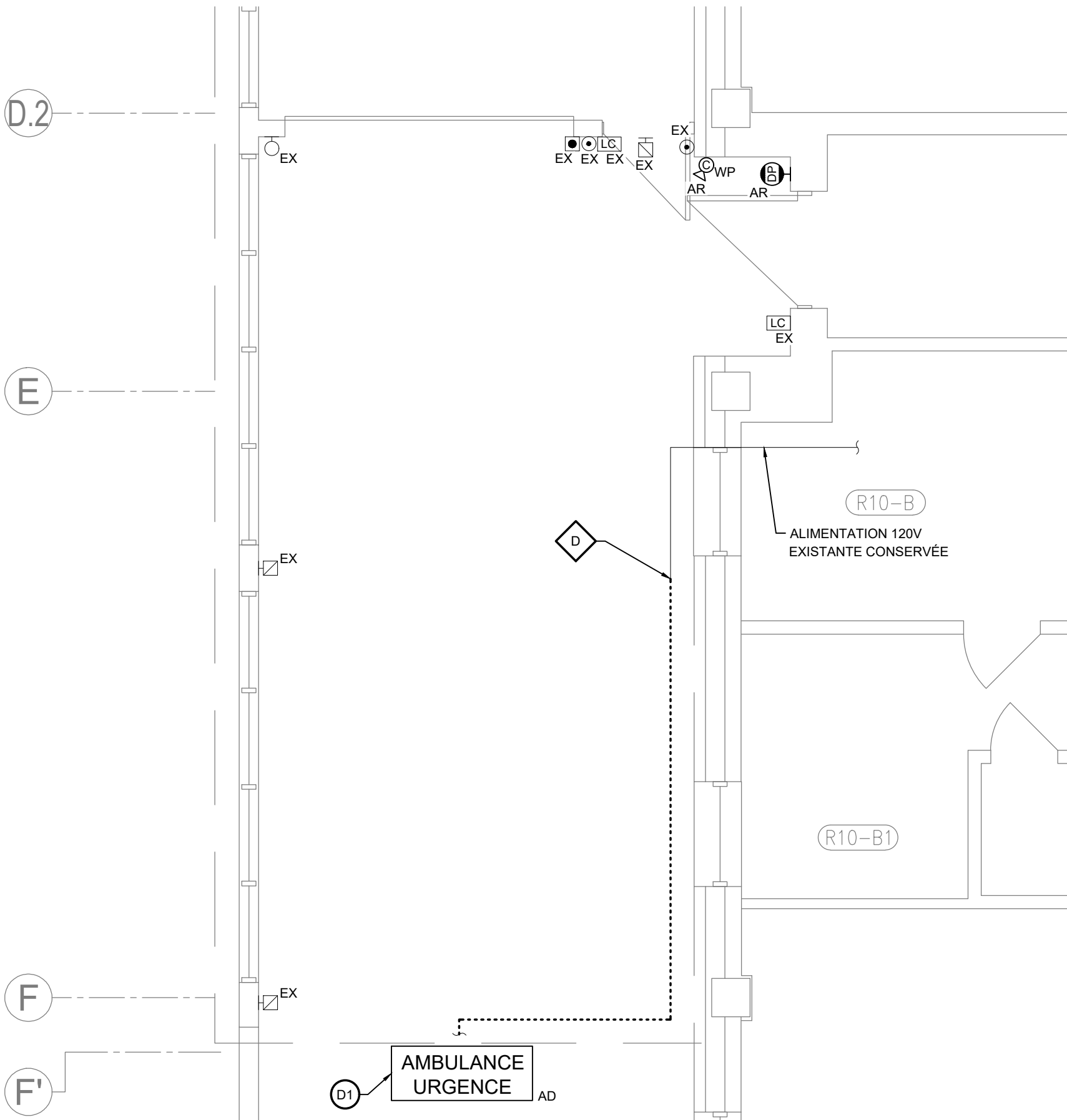
VUE AGRANDIE - QUAI DES AMBULANCES - ÉLECTRICITÉ - DÉMOLITION
