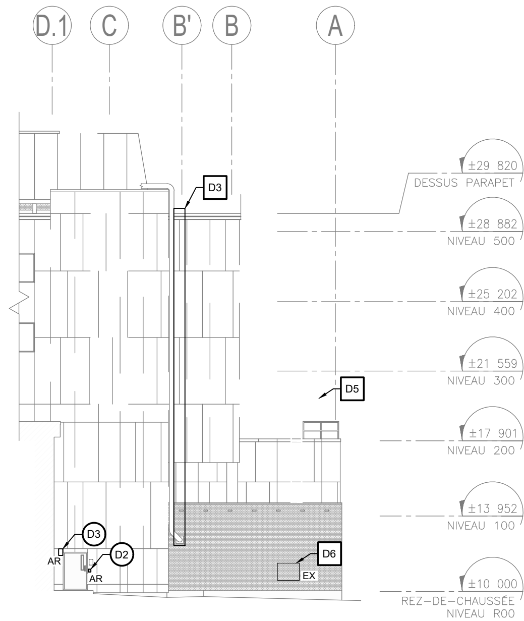
H ÉLÉVATION EST PARTIELLE - DÉMOLITION ÉCHELLE: 1:200
