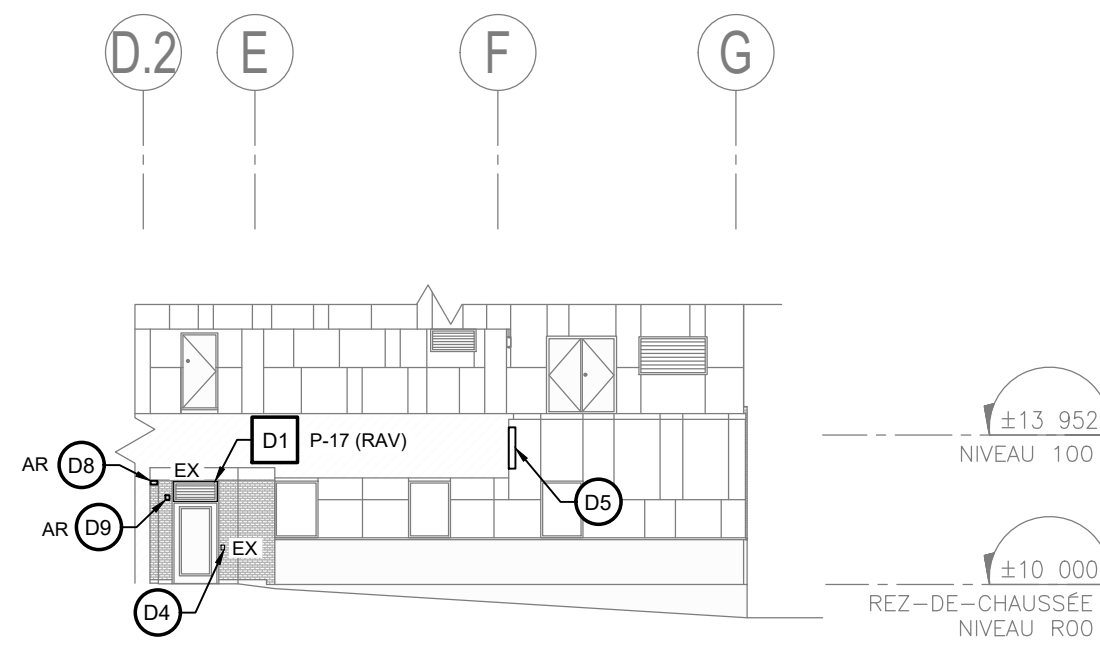
E ÉLÉVATION OUEST PARTIELLE - DÉMOLITION ÉCHELLE: 1:200
