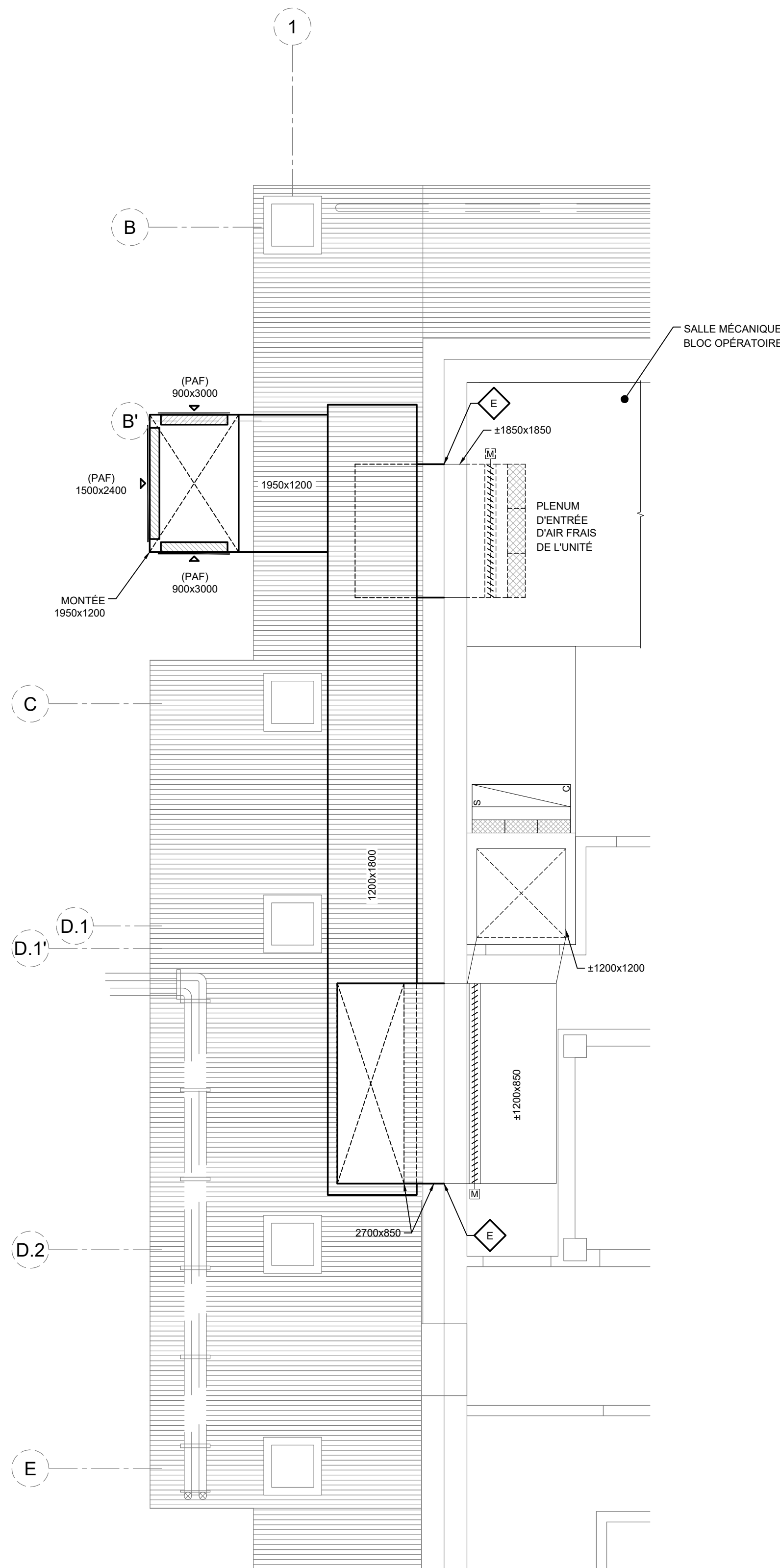
VUE AGRANDIE - TOITURE OUEST - PRISE D'AIR FRAIS BLOC OPÉRATOIRE - CONSTRUCTION
