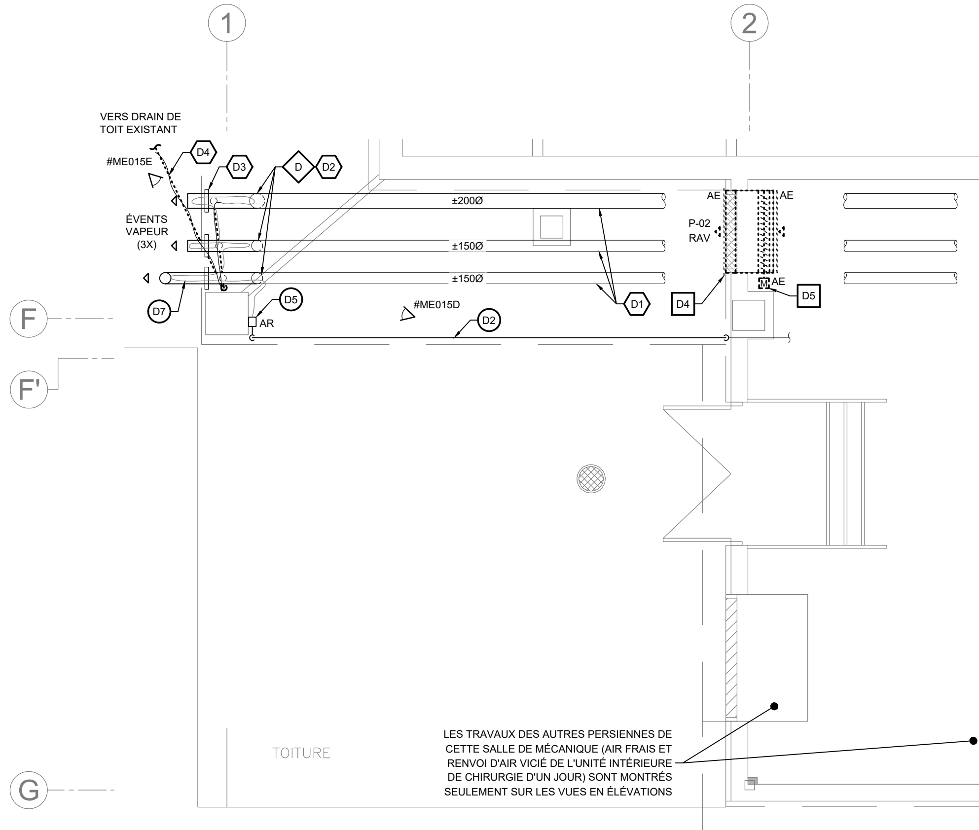
VUE AGRANDIE - SALLE MÉCANIQUE CHIRURGIE D'UN JOUR - DÉMOLITION
