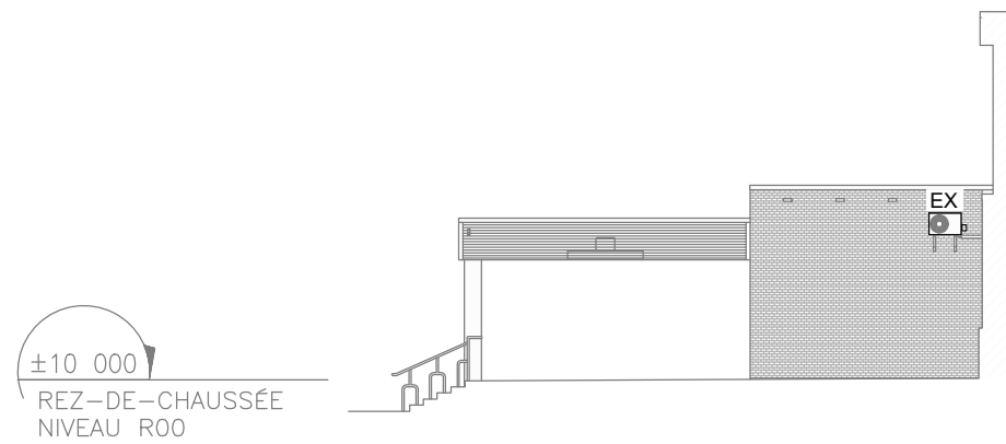
D ÉLÉVATION EST PARTIELLE - CONSTRUCTION ÉCHELLE: 1:200
