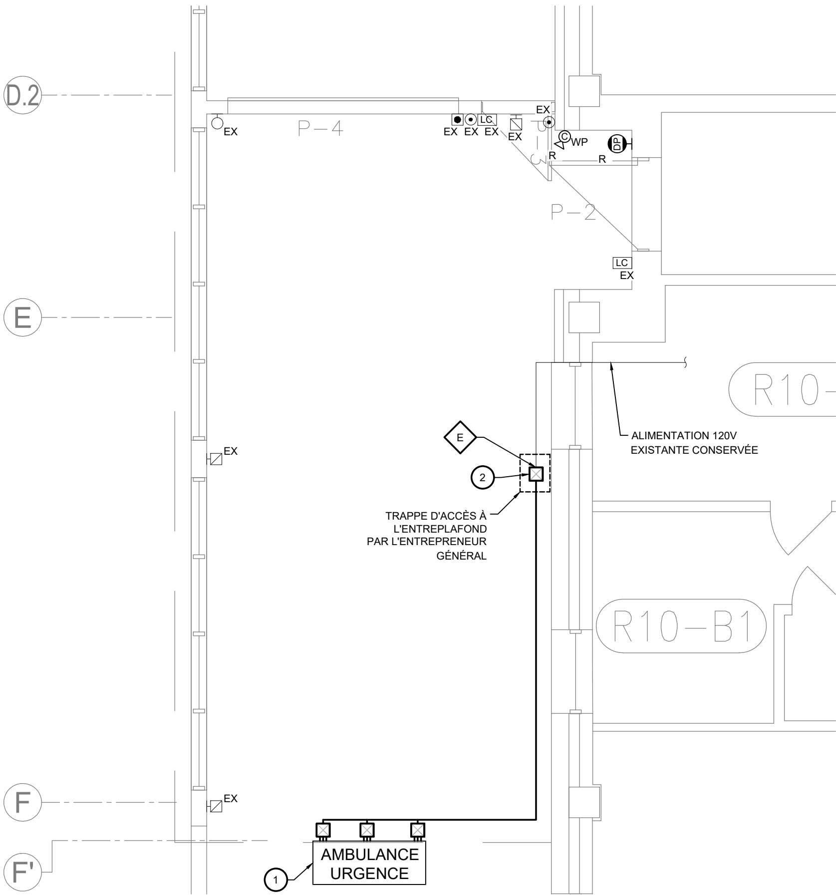
VUE AGRANDIE - QUAI DES AMBULANCES - ÉLECTRICITÉ - CONSTRUCTION
