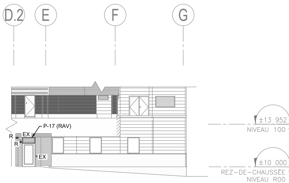
E ÉLÉVATION OUEST PARTIELLE - CONSTRUCTION ÉCHELLE: 1:200
