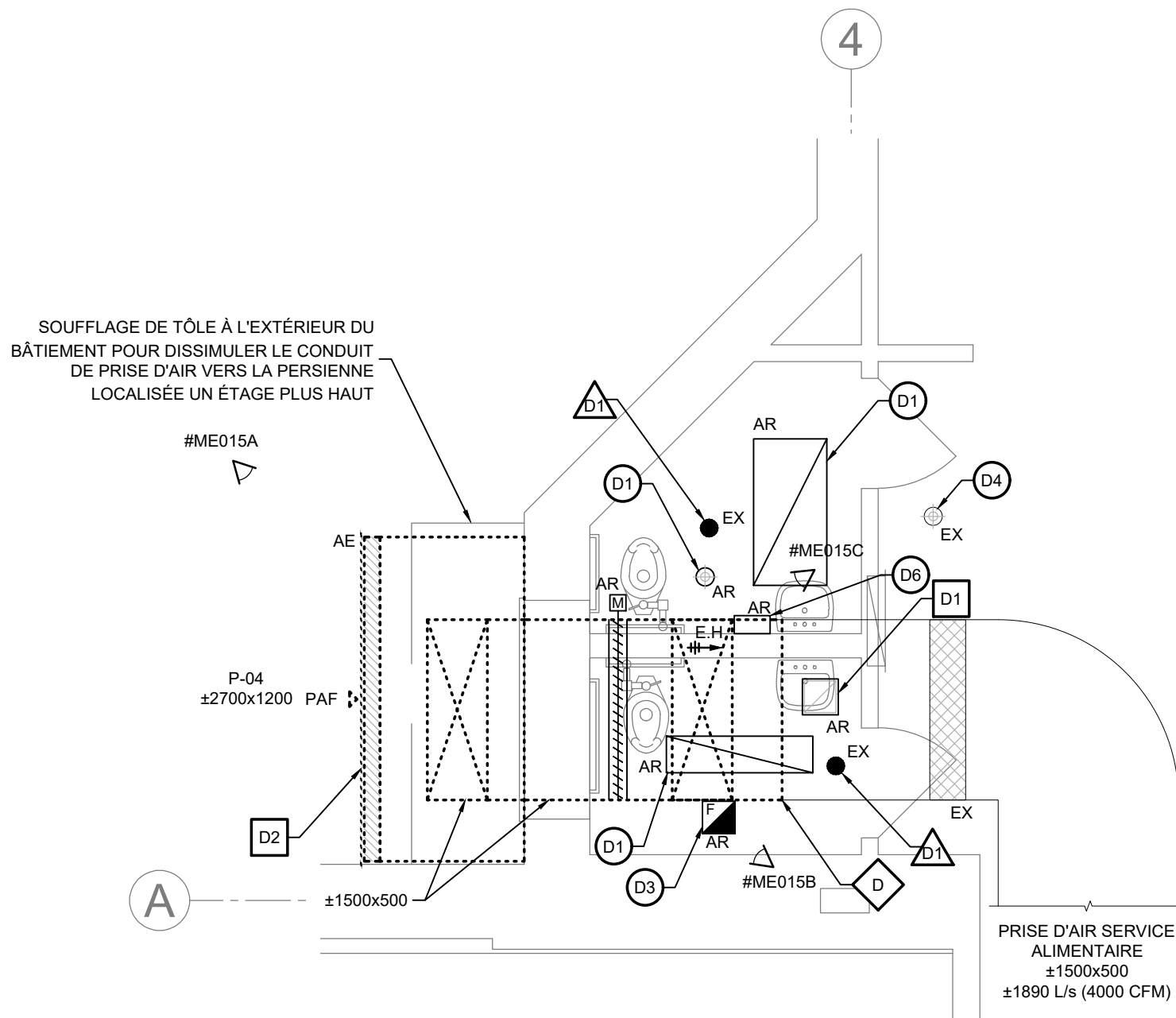
VUE AGRANDIE - PRISE D'AIR SERVICE ALIMENTAIRE - DÉMOLITION
