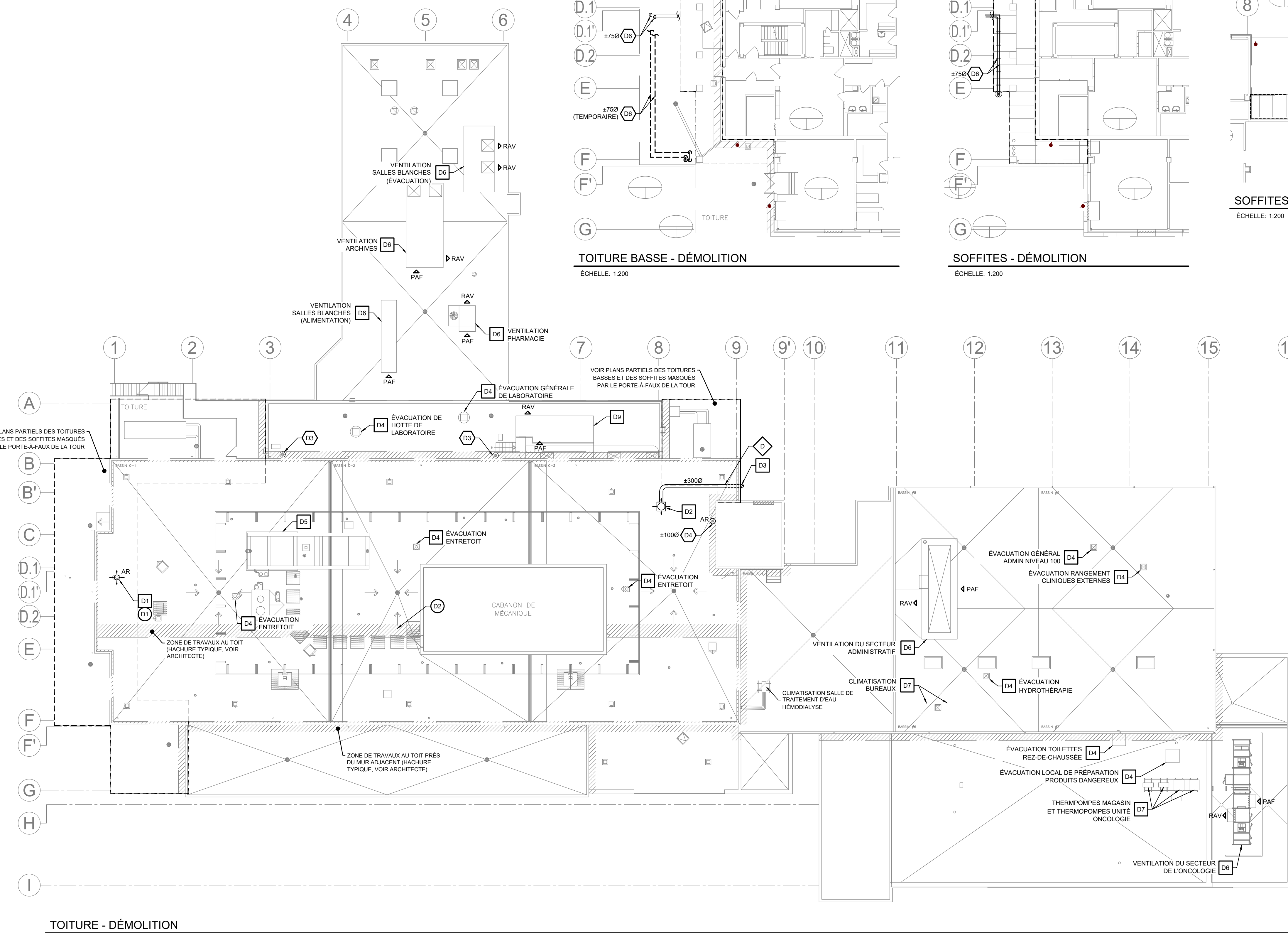
TOITURE - DÉMOLITION
