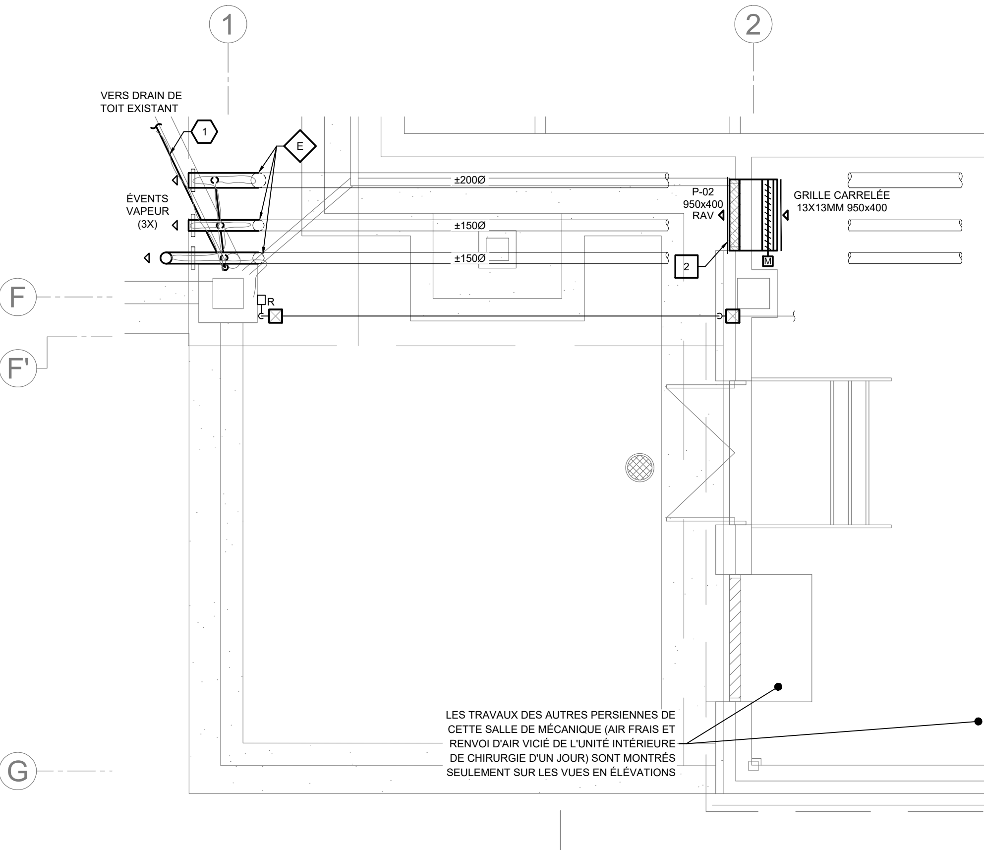
VUE AGRANDIE - SALLE MÉCANIQUE CHIRURGIE D'UN JOUR - CONSTRUCTION
