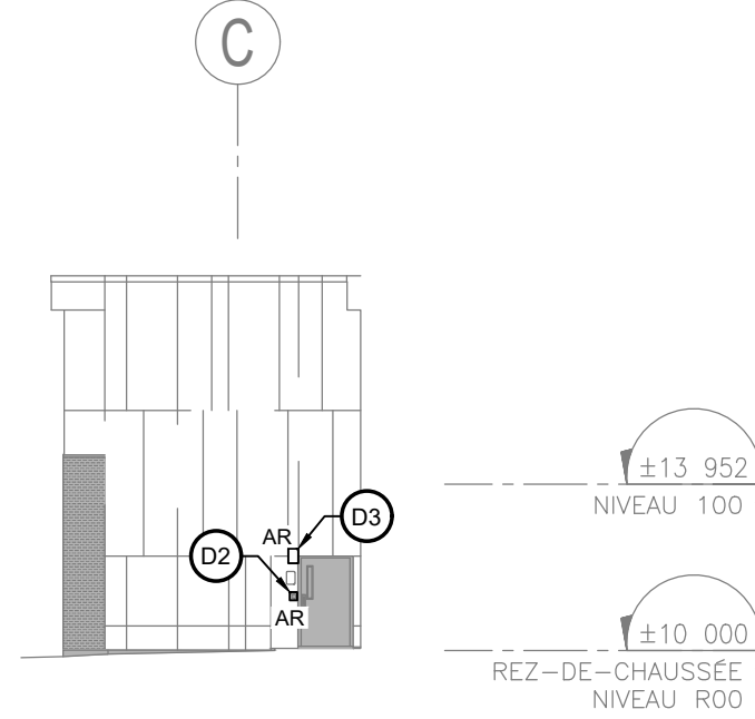
I ÉLÉVATION OUEST PARTIELLE - DÉMOLITION ÉCHELLE: 1:200
