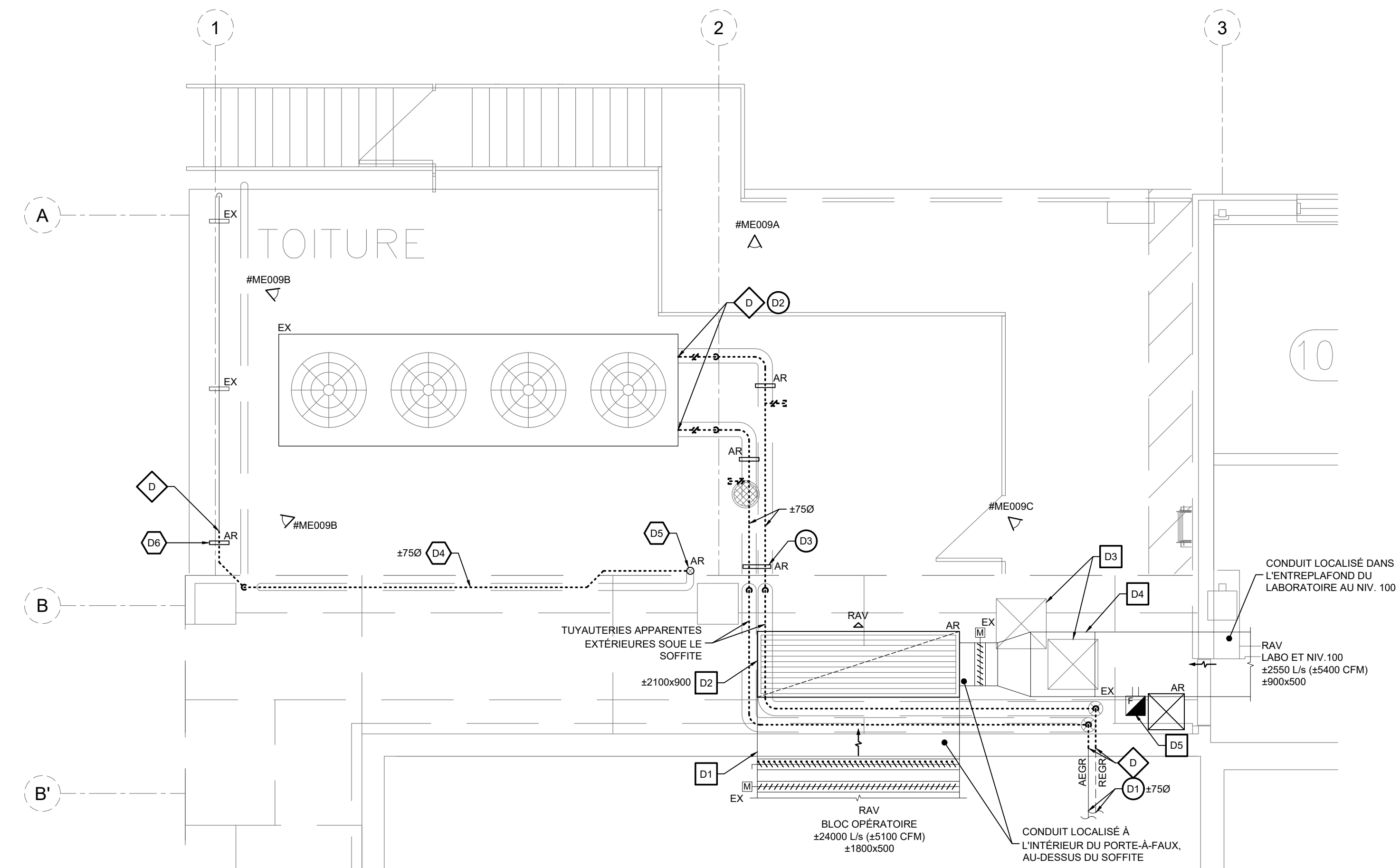
VUE AGRANDIE - TOITURE COIN NORD-OUEST - DÉMOLITION
