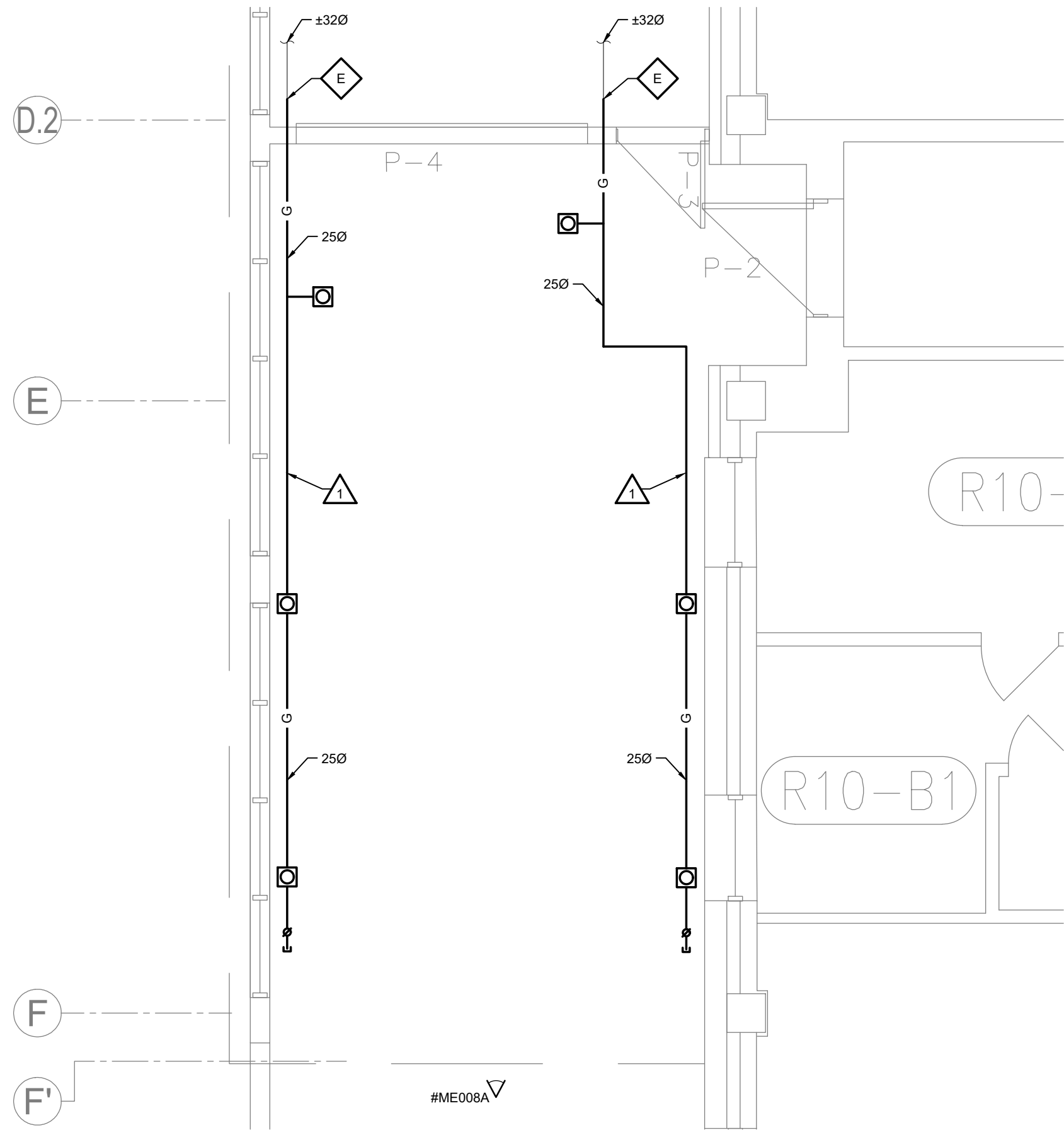
VUE AGRANDIE - QUAI DES AMBULANCES - PROTECTION-INCENDIE - CONSTRUCTION
