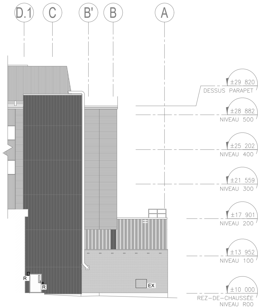
H ÉLÉVATION EST PARTIELLE - CONSTRUCTION ÉCHELLE: 1:200
