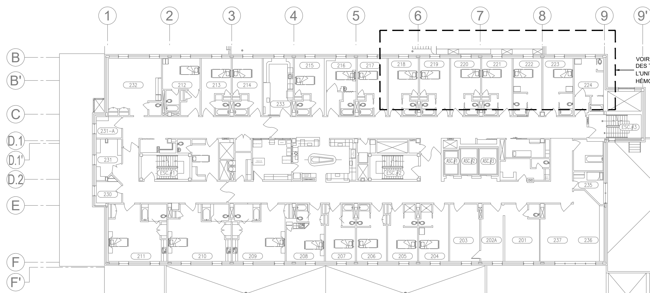
ÉCHELLE: 1:250
