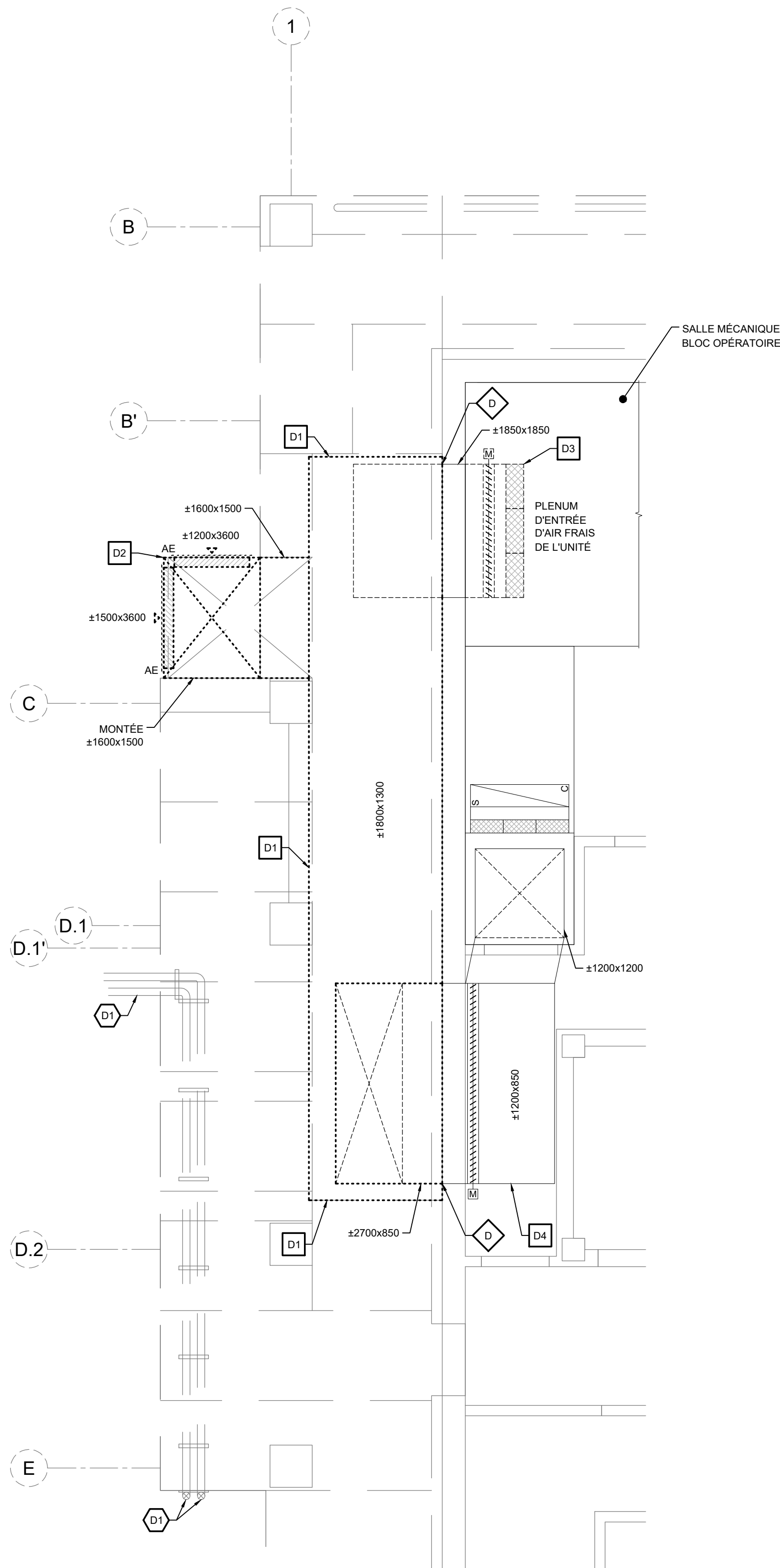
VUE AGRANDIE - TOITURE OUEST - PRISE D'AIR FRAIS BLOC OPÉRAIRE - DÉMOLITION
