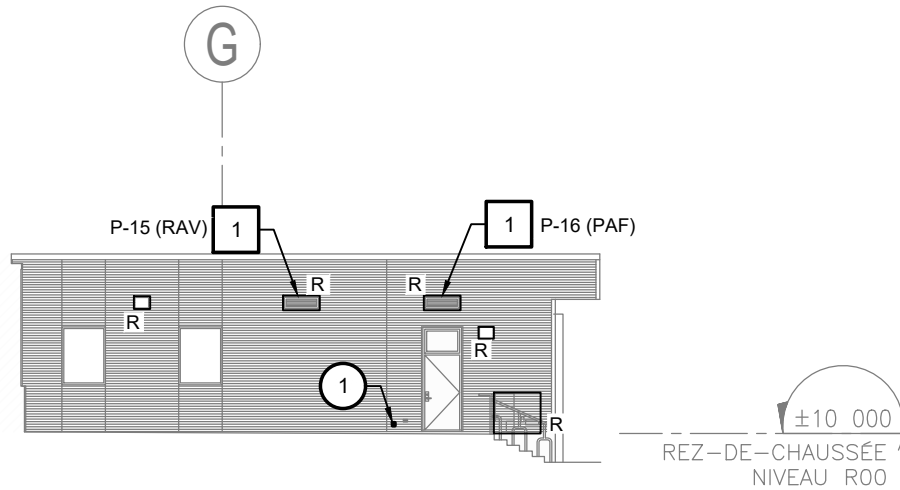
C ÉLÉVATION OUEST PARTIELLE - CONSTRUCTION ÉCHELLE: 1:200
