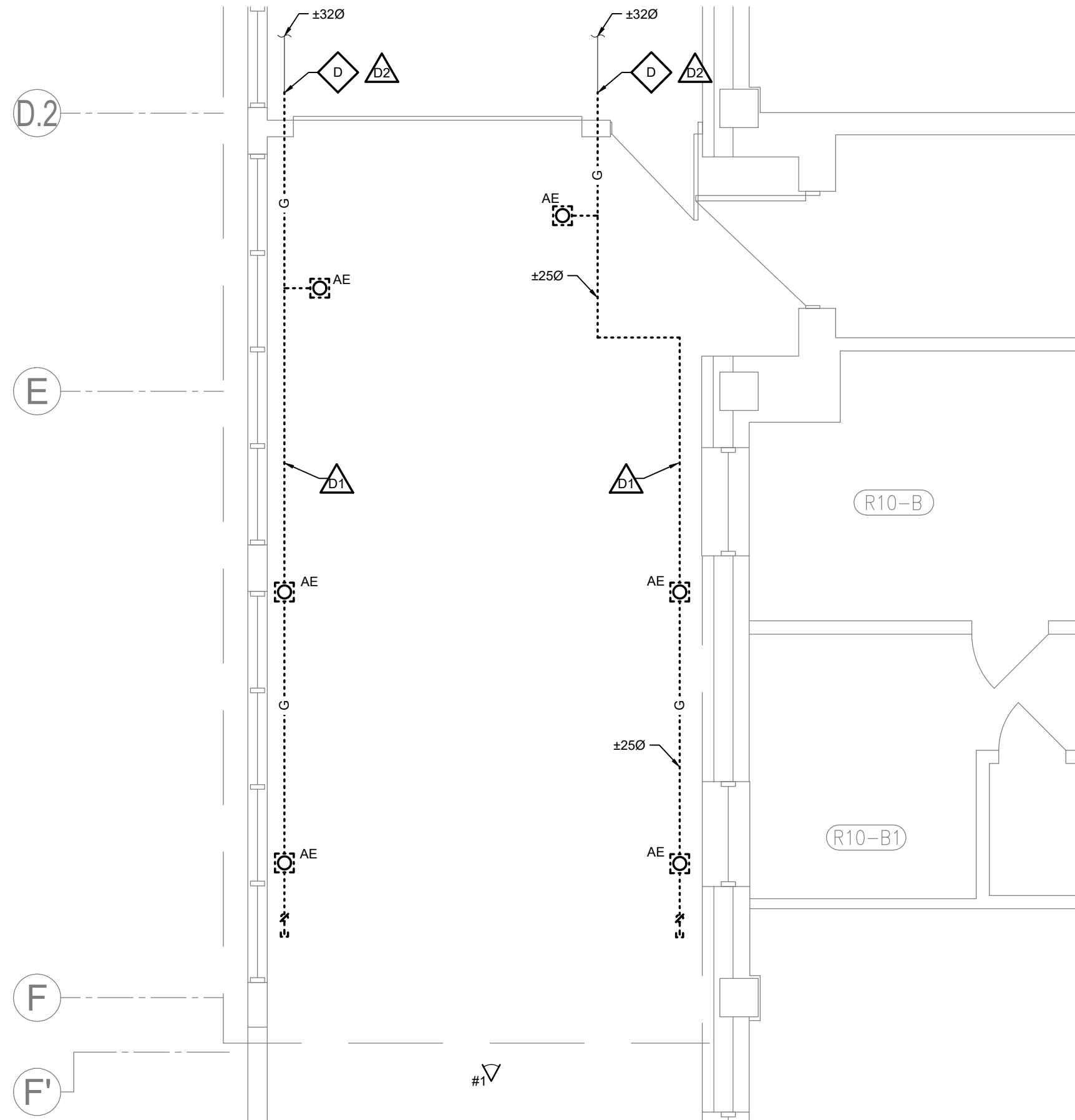
VUE AGRANDIE - QUAI DES AMBULANCES - PROTECTION-INCENDIE - DÉMOLITION
