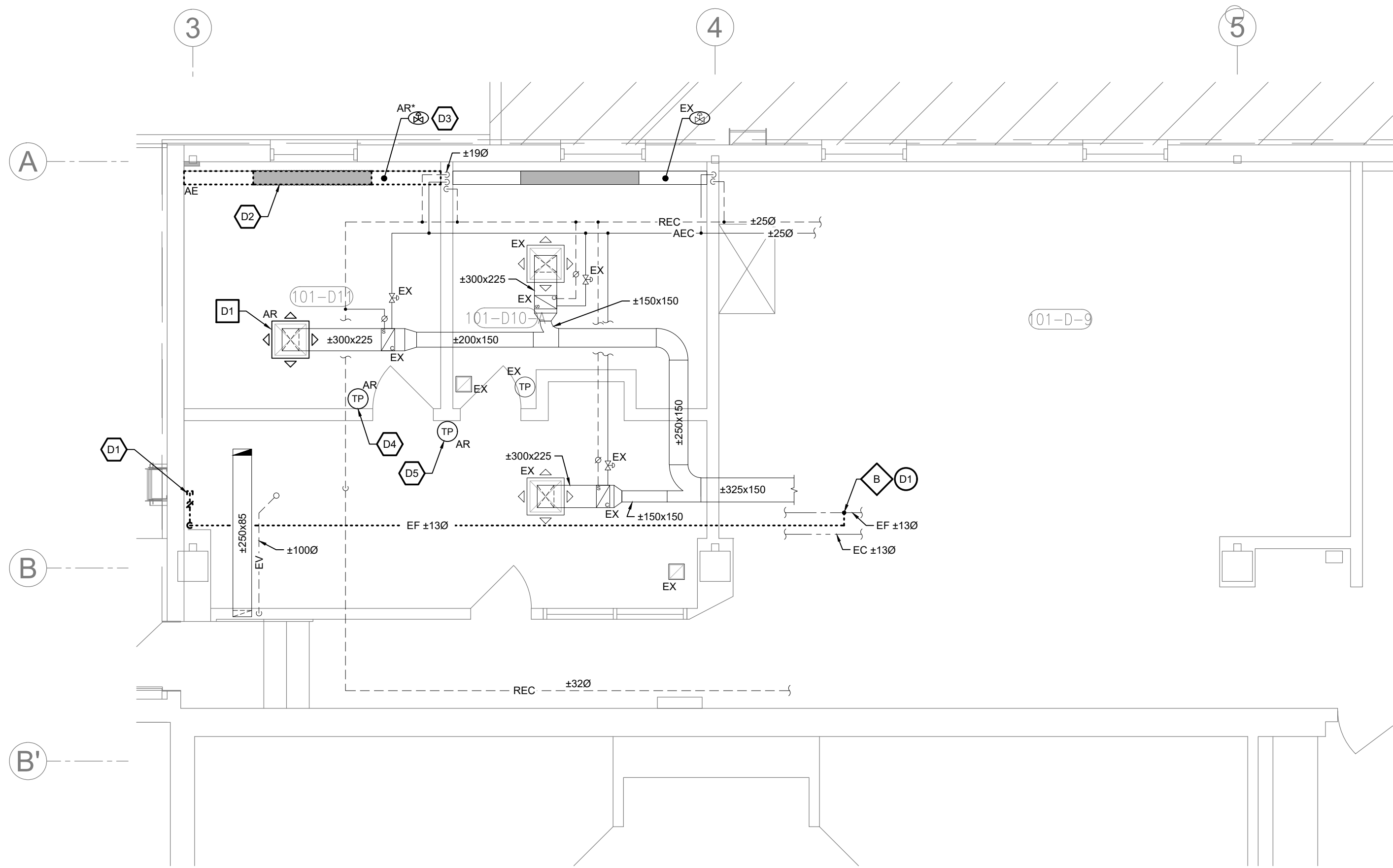
VUE AGRANDIE - AJOUT ISSUE LABORATOIRE - MÉCANIQUE - DÉMOLITION
