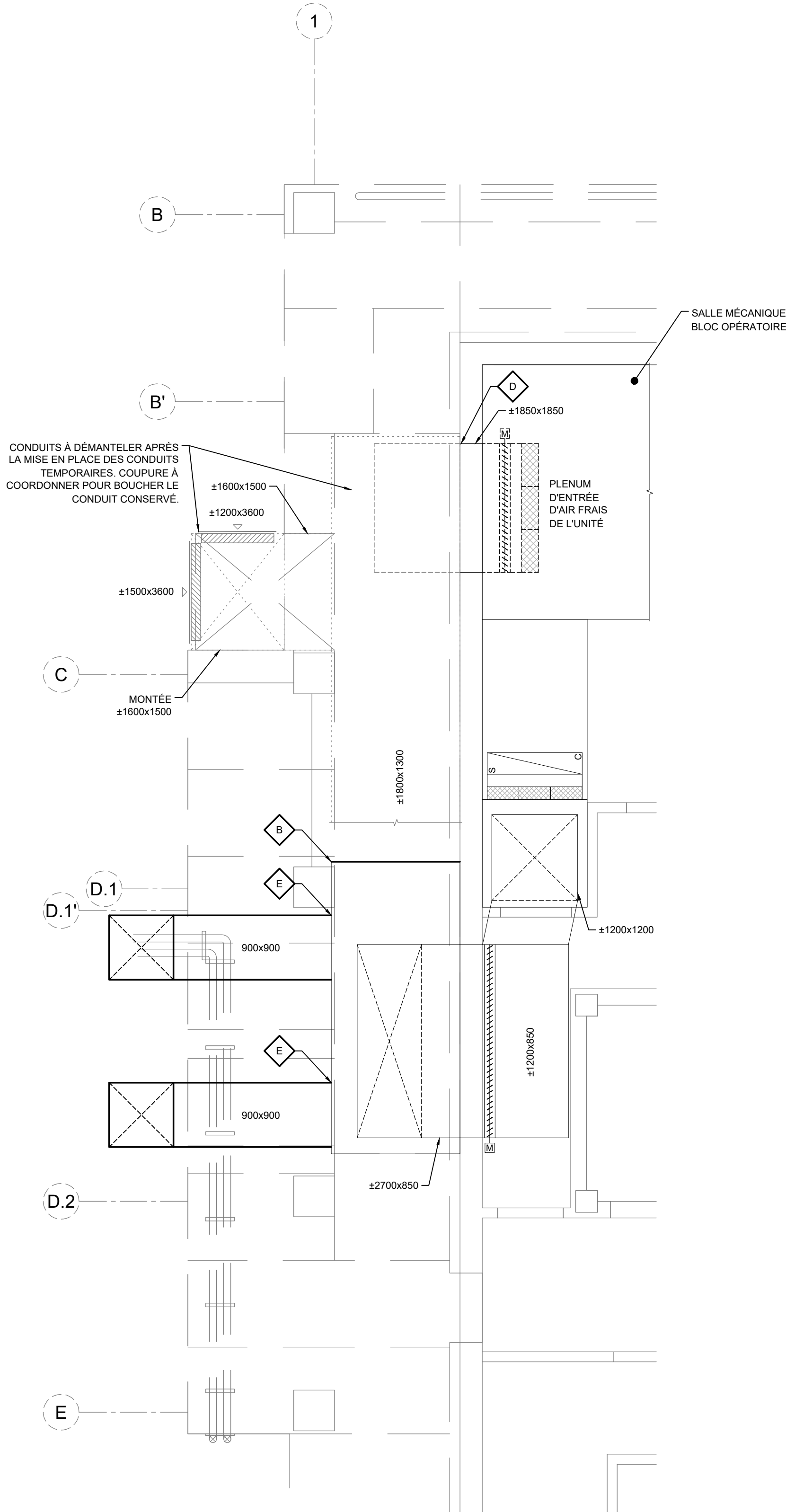
VUE AGRANDIE - TOITURE OUEST - PRISE D'AIR FRAIS BLOC OPÉRATEIRE - TEMPORAIRE #1
