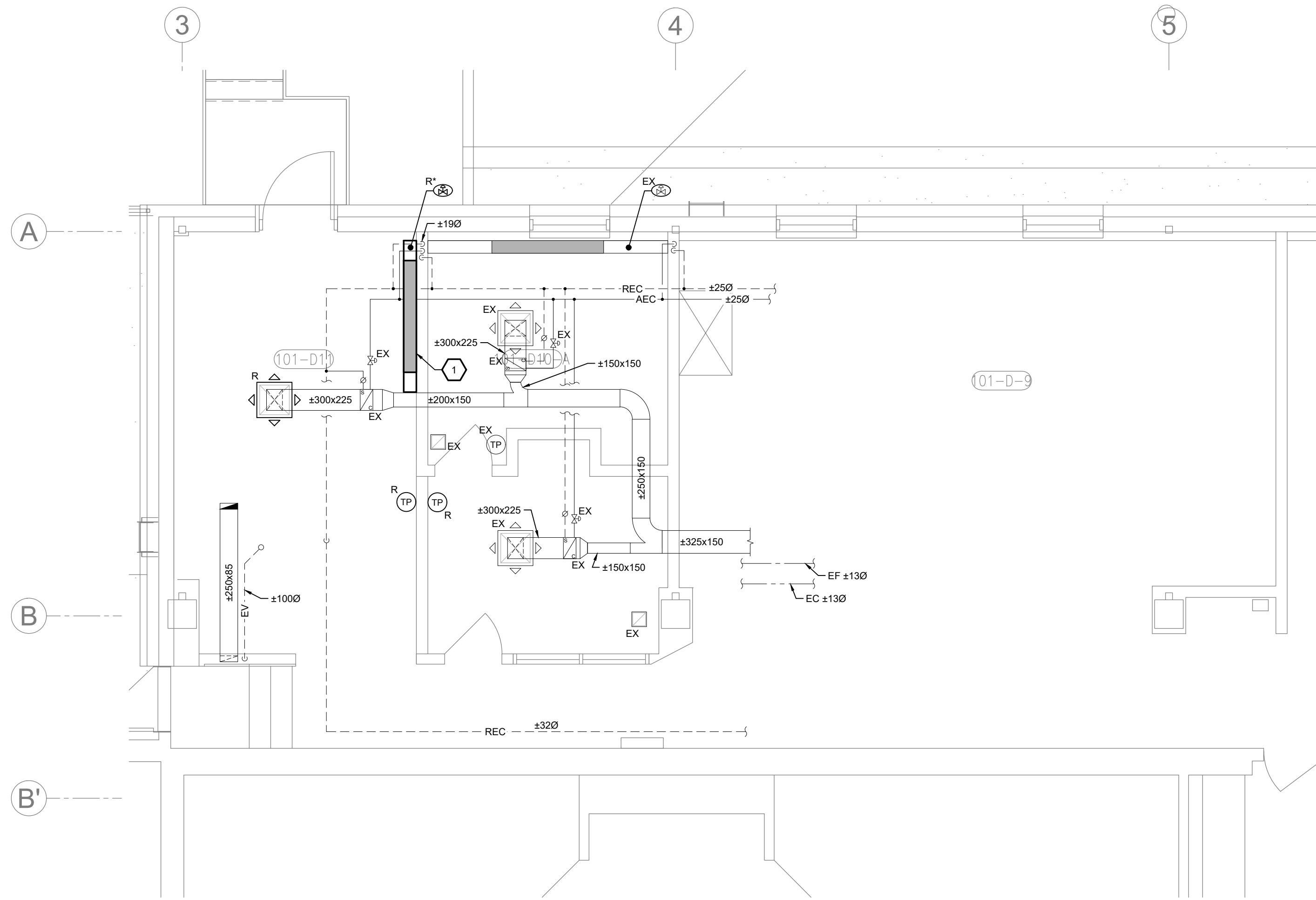
VUE AGRANDIE - AJOUT ISSUE LABORATOIRE - MÉCANIQUE - CONSTRUCTION
